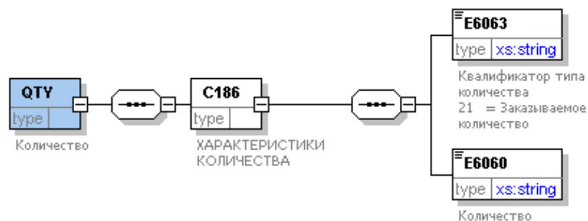
Рисунок 14 –Диаграмма соответствующего сегменту QTY одноименного элемента данных QTY в синтаксисе XML
