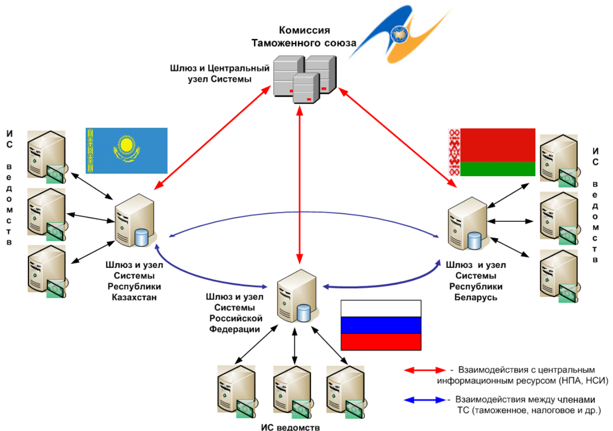
Рис 1. Архитектура Системы
